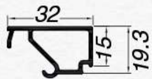
22.4532 junquillo 32 mm hueco 39 mm BP
