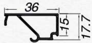
22.4536 junquillo 36 mm hueco 35 mm
