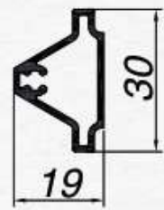
22.3800 - pletina travesaño BP
