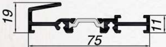
22.6003 - solera ML (barras de 3,5 m) BP
