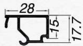
22.4528 junquillo 28 mm hueco 43 mm BP
