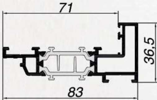
22.6511 - acople apertura exterior BP
