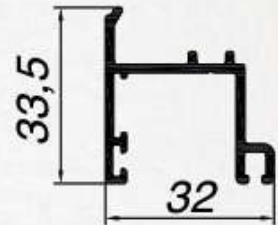
22.6000 - vierteaguas hoja (barras de 3,5 m)
