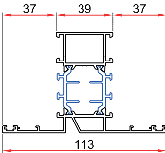
90.3977 TRAVESAÑO
