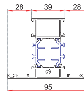
90.3978 TRAVESAÑO
