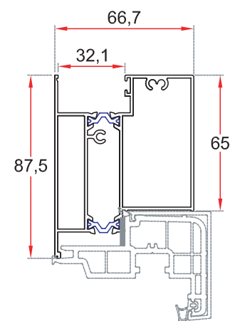
79.2236 TRAVESAÑO HOJA
