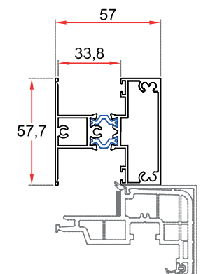
79.2436 TRAVESAÑO HOJA
