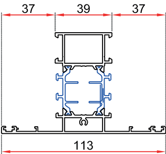
90.3976 TRAVESAÑO
