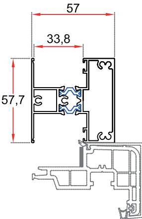
79.2436 TRAVESAÑO HOJA
