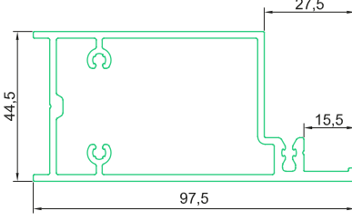
20.2201 FULLA CORREDISSA
