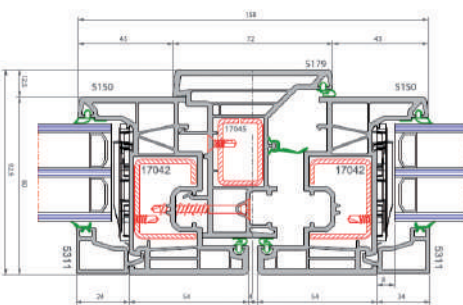
SECCIÓ HORIZONTAL
