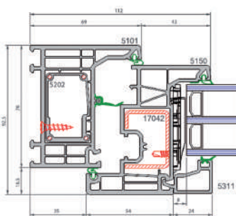
SECCIÓ VERTICAL
