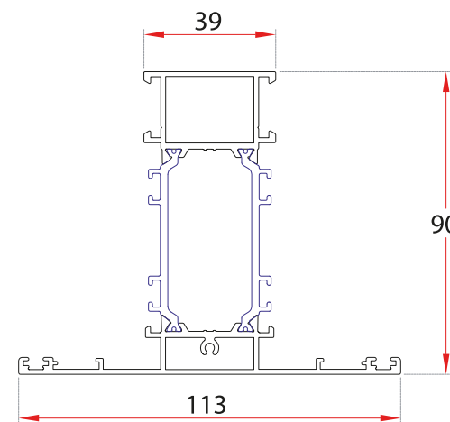
89.3980 TRAVESAÑO
