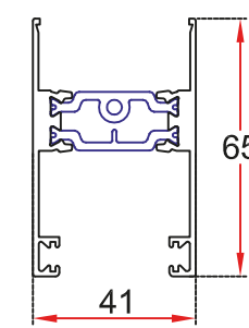
78.2270 CASACA
