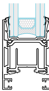
78.2170 HOJA LATERAL
