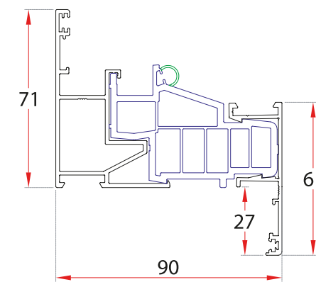
89.1141 MASOLAPE 27
